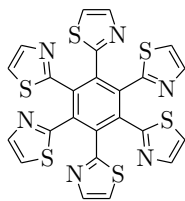
④ ディスク状 6 座配位子
