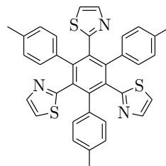
⑤ ディスク状 3 座配位子
