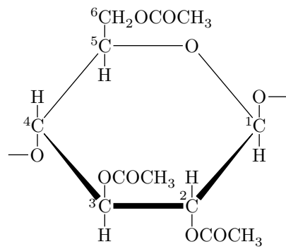
トリアセチルセルロース繰り返し単位
