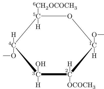
ジアセチルセルロース繰り返し単位
