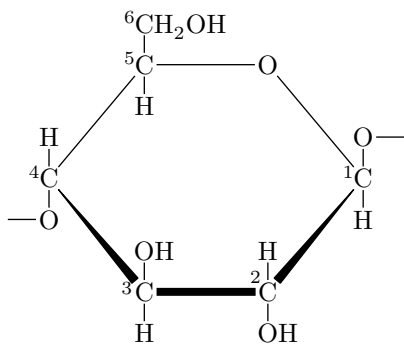
セルロース繰り返し単位
